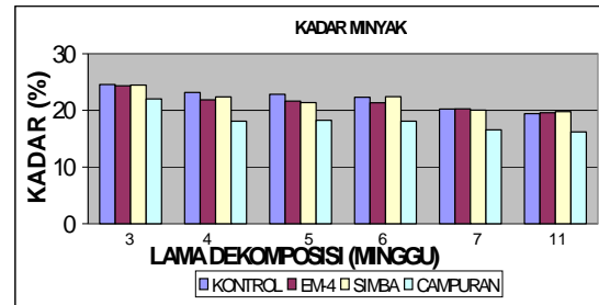
Gambar 3. Penurunan komponen minyak mulai minggu 3 s.d. 11 pada proses dekomposisi limbah bungkil biji jarak
