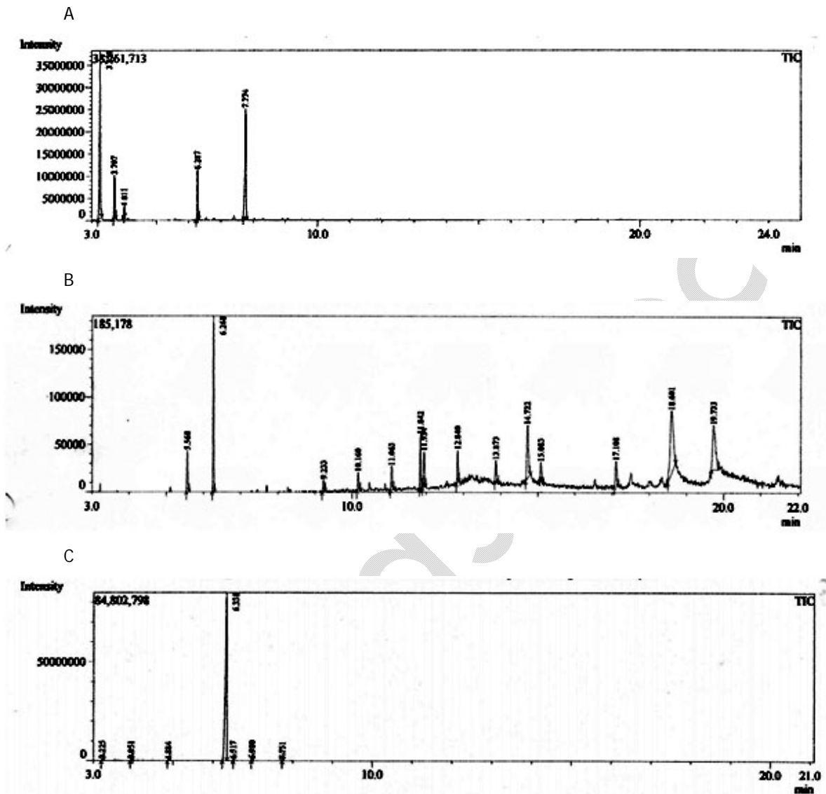
Gambar 1. Kromatogram hasil Gas Chromatography-Mass Spectrometer (GC-MS) dari minyak atsiri yang terkandung dalam: (A) daun kapas yang telah terinfestasi oleh A. biguttulla , (B) Batang dan daun jagung, dan (C) Daun teh hitam.
